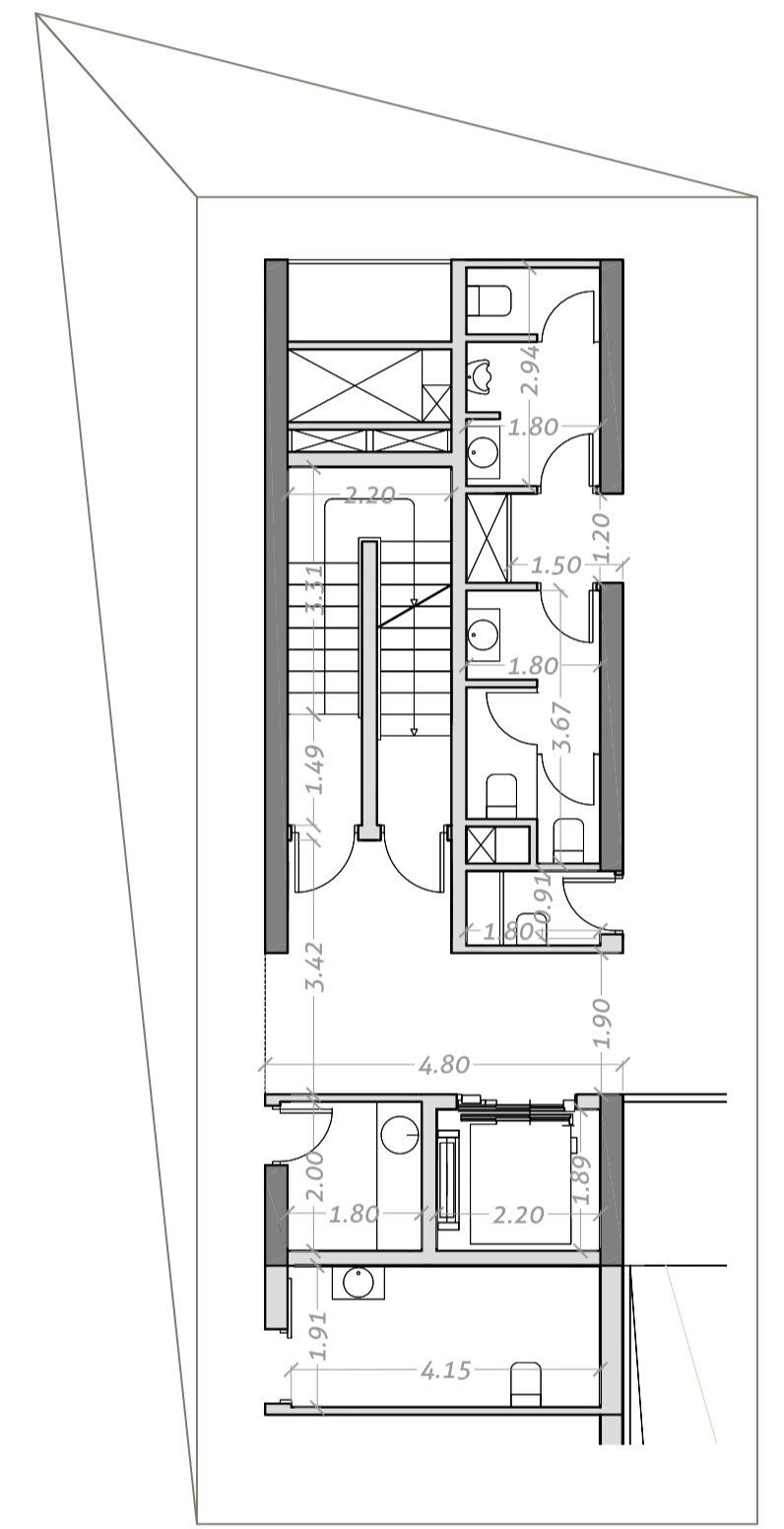
Núcleo de los módulos A, B y C E 1:100
