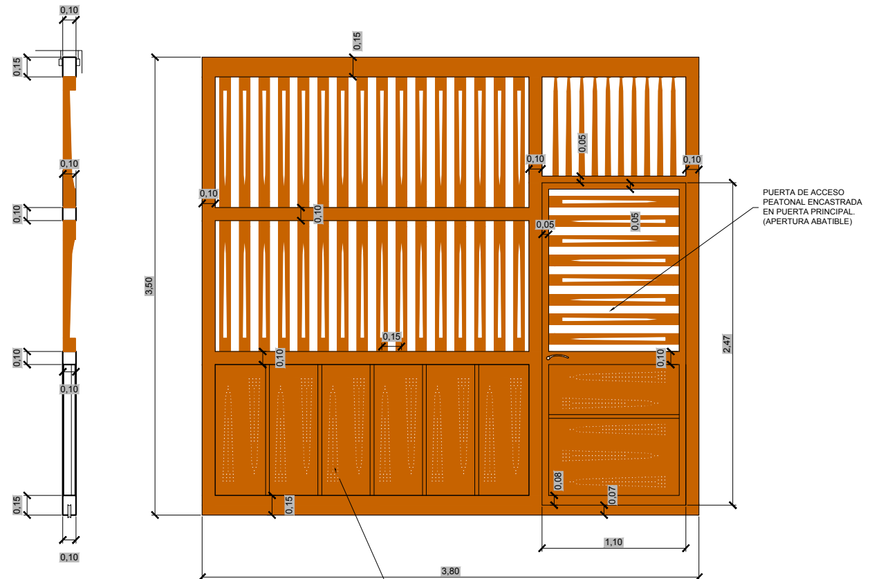
1 HOJA DE PUERTA DE CORREDERA TIPO. HUECO A SALVAR: 6.00m
