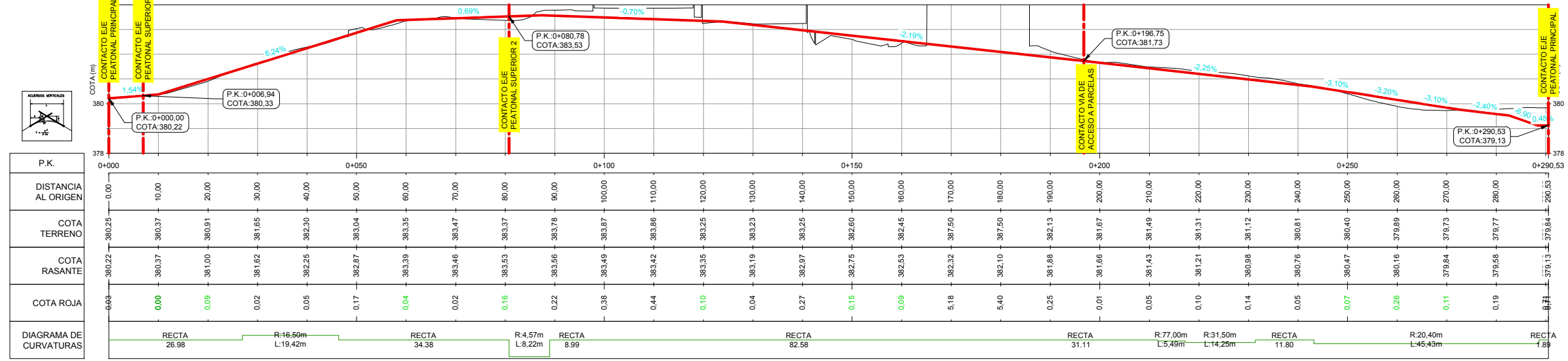
Perfil Longitudinal: PEATONAL SUPERIOR-1 Escala - V: 100 H:500
