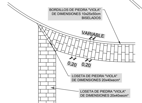
DETALLE PAVIMENTO EN ENCUENTROS RECTA-CURVA ESC.: 1:50
