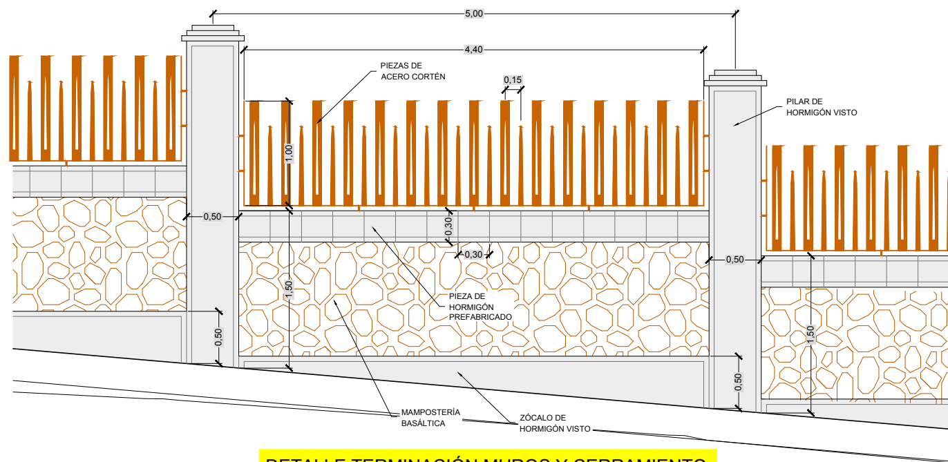
DETALLE TERMINACIÓN MUROS Y CERRAMIENTO EN CAMINO LAS MANTECAS ESC. 1:25
