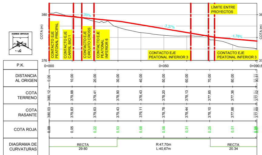
Perfil Longitudinal: PEATONAL INFERIOR-2 Escala - V: 100 H:500
