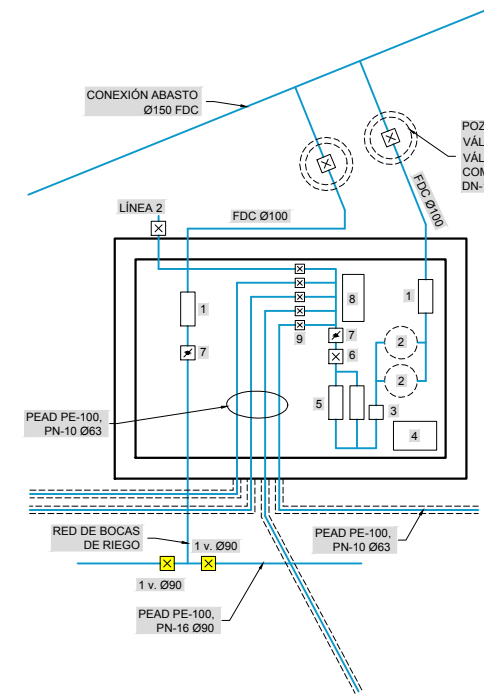
CROQUIS INSTALACIONES EN CABEZAL DE RIEGO
